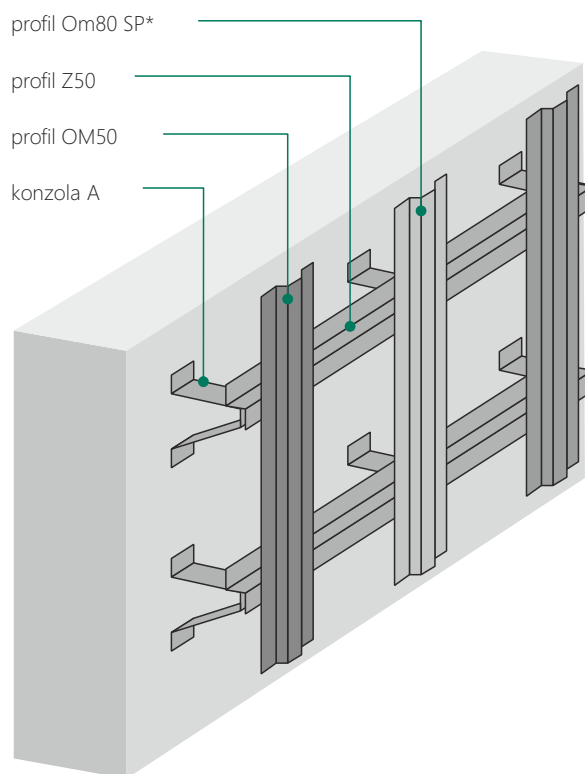
rošt DKM2A
