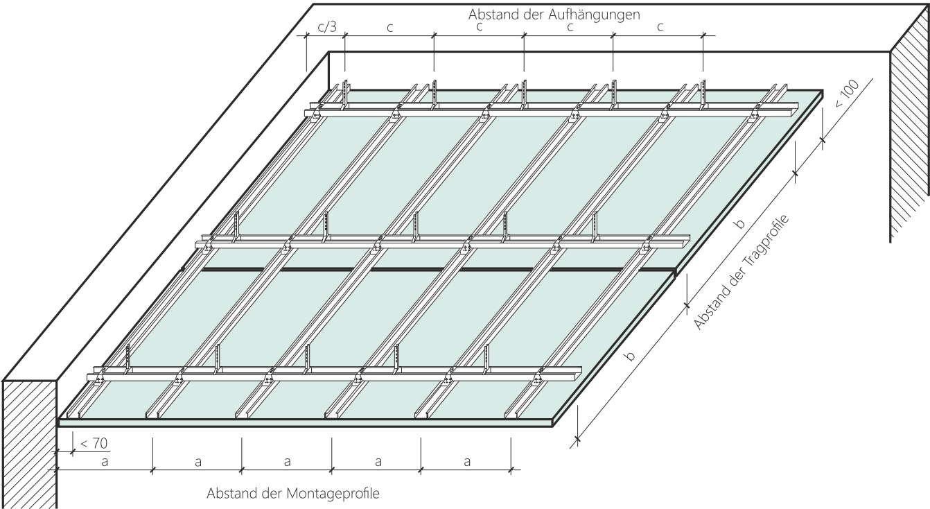
Schema der tragenden Konstruktion der Untersicht fr die Verkleidung mit zementgebundener Spanplatte CETRIS® (Dicke 12 mm)
