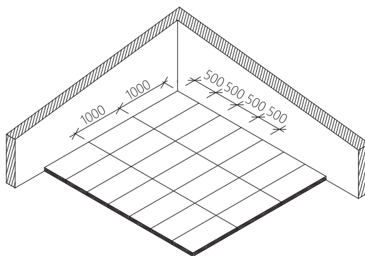
Kladení izolačních desek
