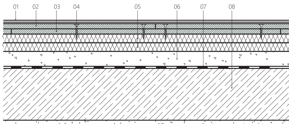
Vyrovnání nerovného podkladu, zvýšení konstrukční výšky IZOCET - svislý řez
