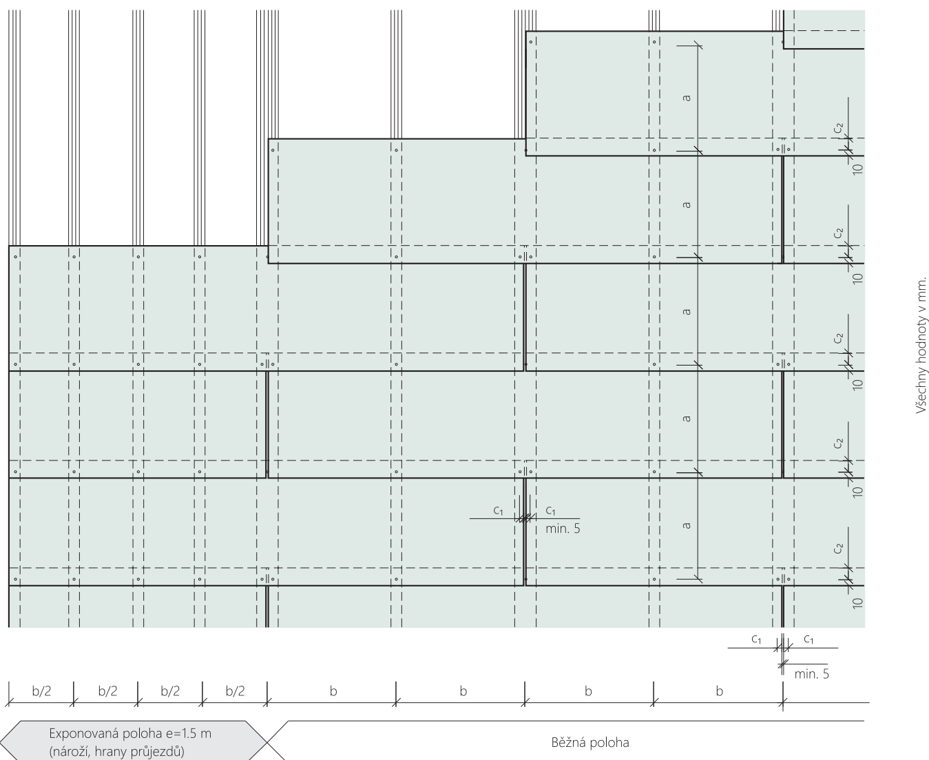
Schéma uložení desek CETRIS® PLANK
