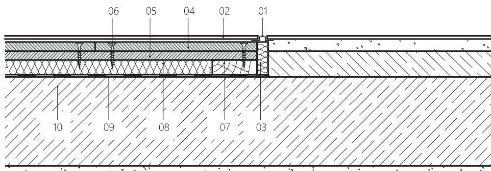
Přechod na jinou podlahu IZOCET - svislý řez
