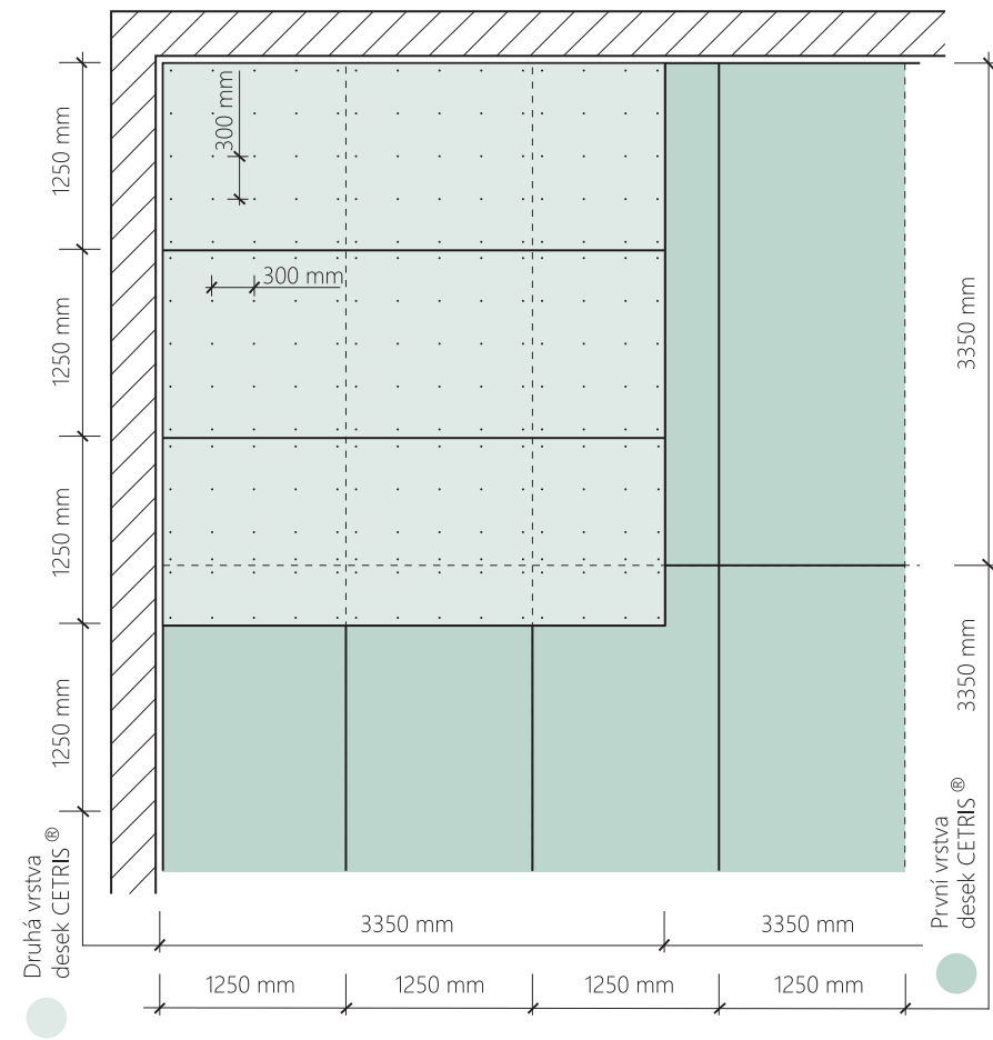
Kladení desek CETRIS® formátu 1250 x 3350 mm - plovoucí podlahy IZOCET, POLYCET
