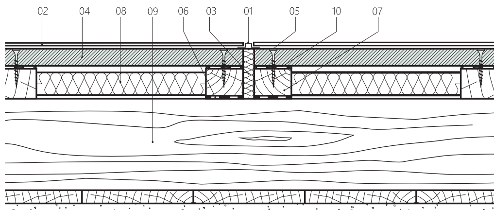
Podlahové desky na nosnících – řešení dilatace
