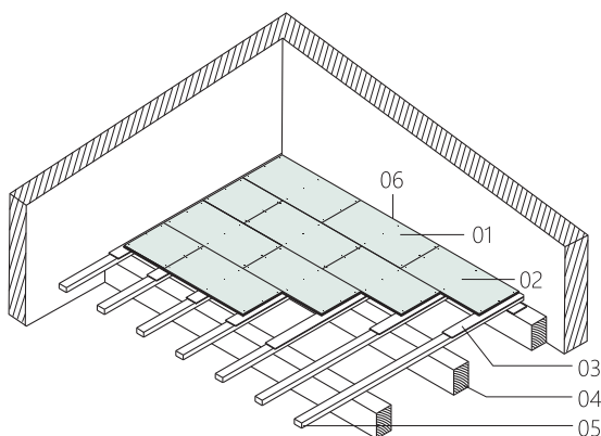
Podlahové desky na nosnících – postup pokládání
