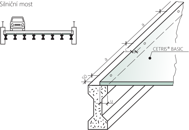
Silniční most
