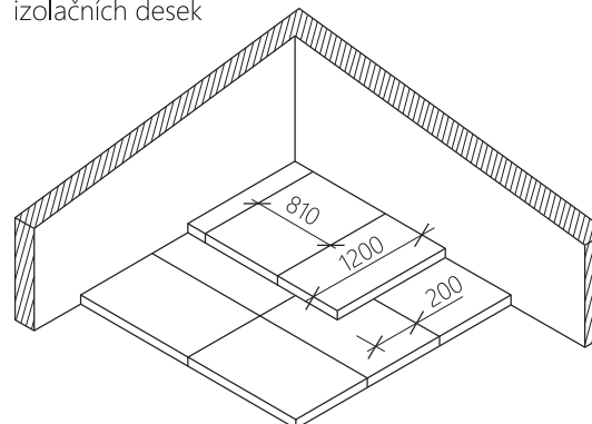
Kladení druhé vrstvy izolačních desek
