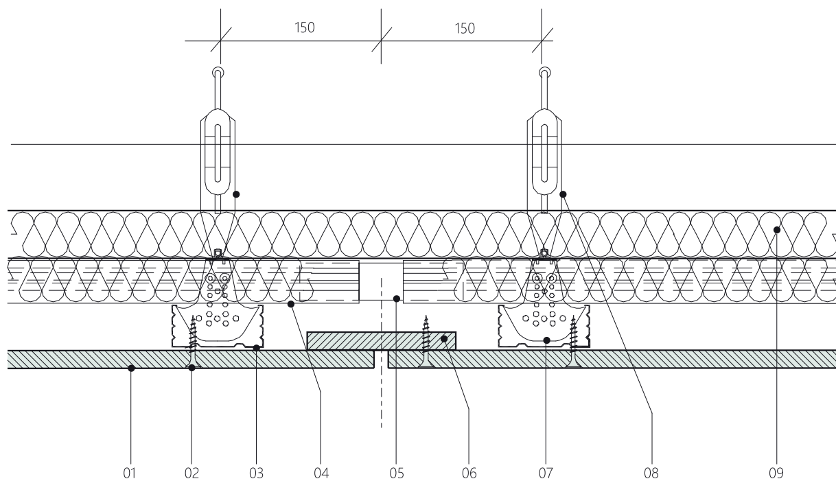
Dilatační spára v pohledu
