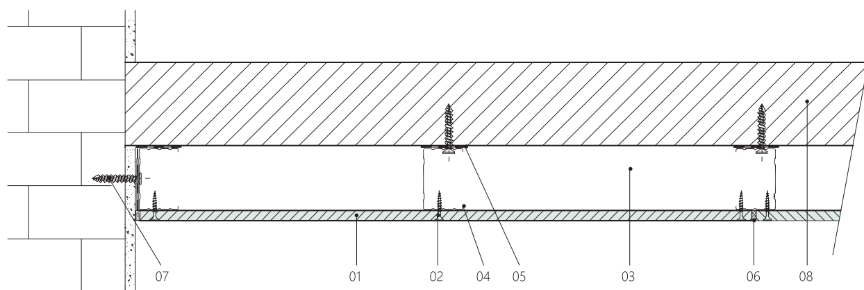
Napojení u stěny - Vodorovný řez
