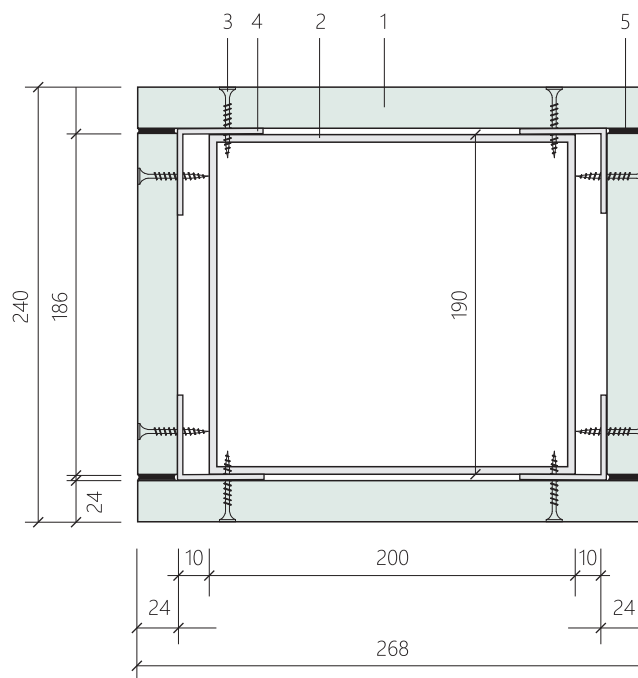
b) obklad pravoúhlých uzavřených profilů
