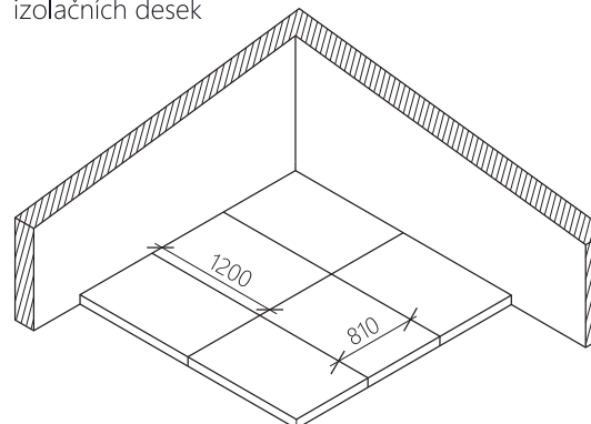
Kladení první vrstvy izolačních desek
