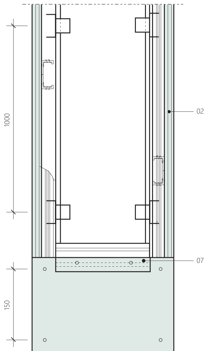
Svislý řez
