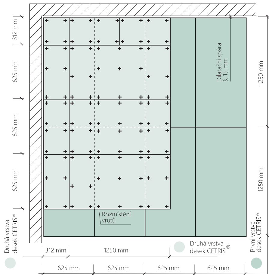
Kladení desek CETRIS® formátu 1250 x 3350 mm - plovoucí podlahy IZOCET, POLYCET
