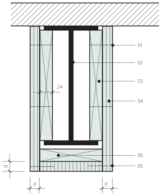
Příčný řez
