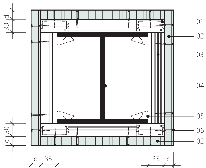
Vodorovný řez
