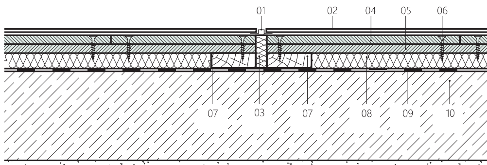
Dilatační spára v ploše IZOCET - svislý řez
