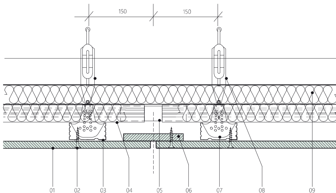
Dilatační spára v pohledu
