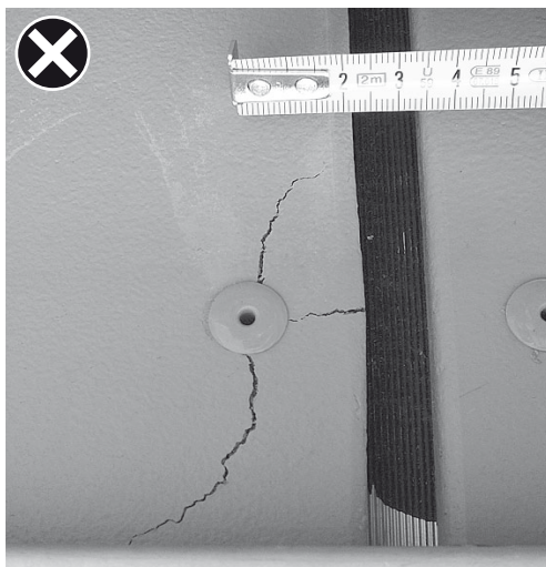
Nedostatečný odstup krajního nýtu
