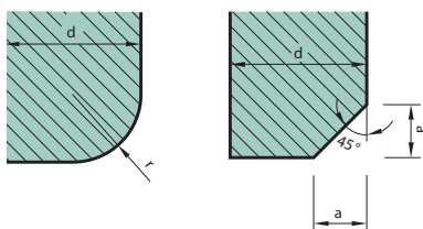
Sražení hran pro desky CETRIS® v systému PLANK
